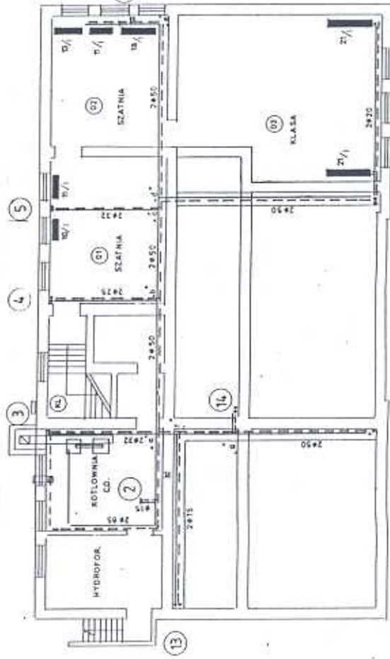
Rzut piwnic - dziś mieszczących m.in. szatnie i pracownię
