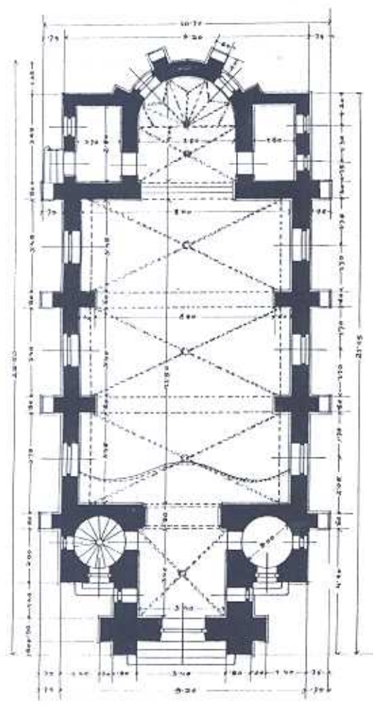
Rzut przyziemia kościoła zaprojektowanego dla Tamawic przez J. Nikodemowicza w roku 1912
